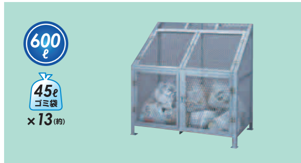
CS-07 ダストBOX 1200mm ・溶融亜鉛メッキ ●サイズ/(約)W1200×D700×H1200mm ●重量/(約)64kg ●JAN/4990127 006251
